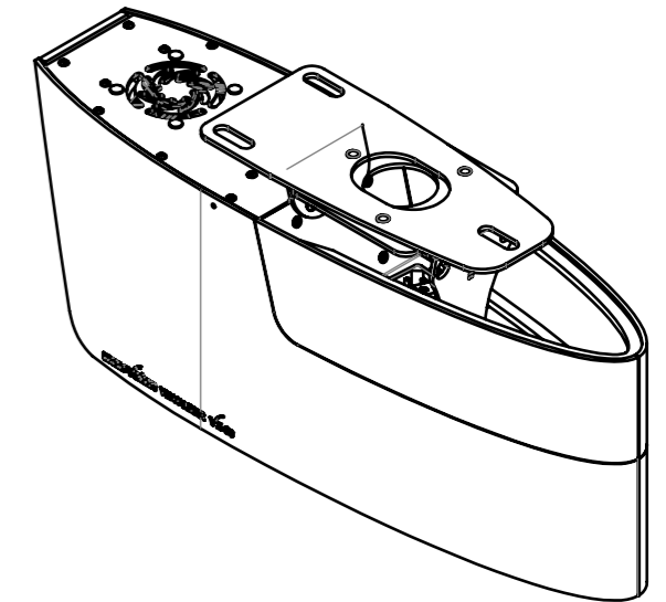
M 1:5
